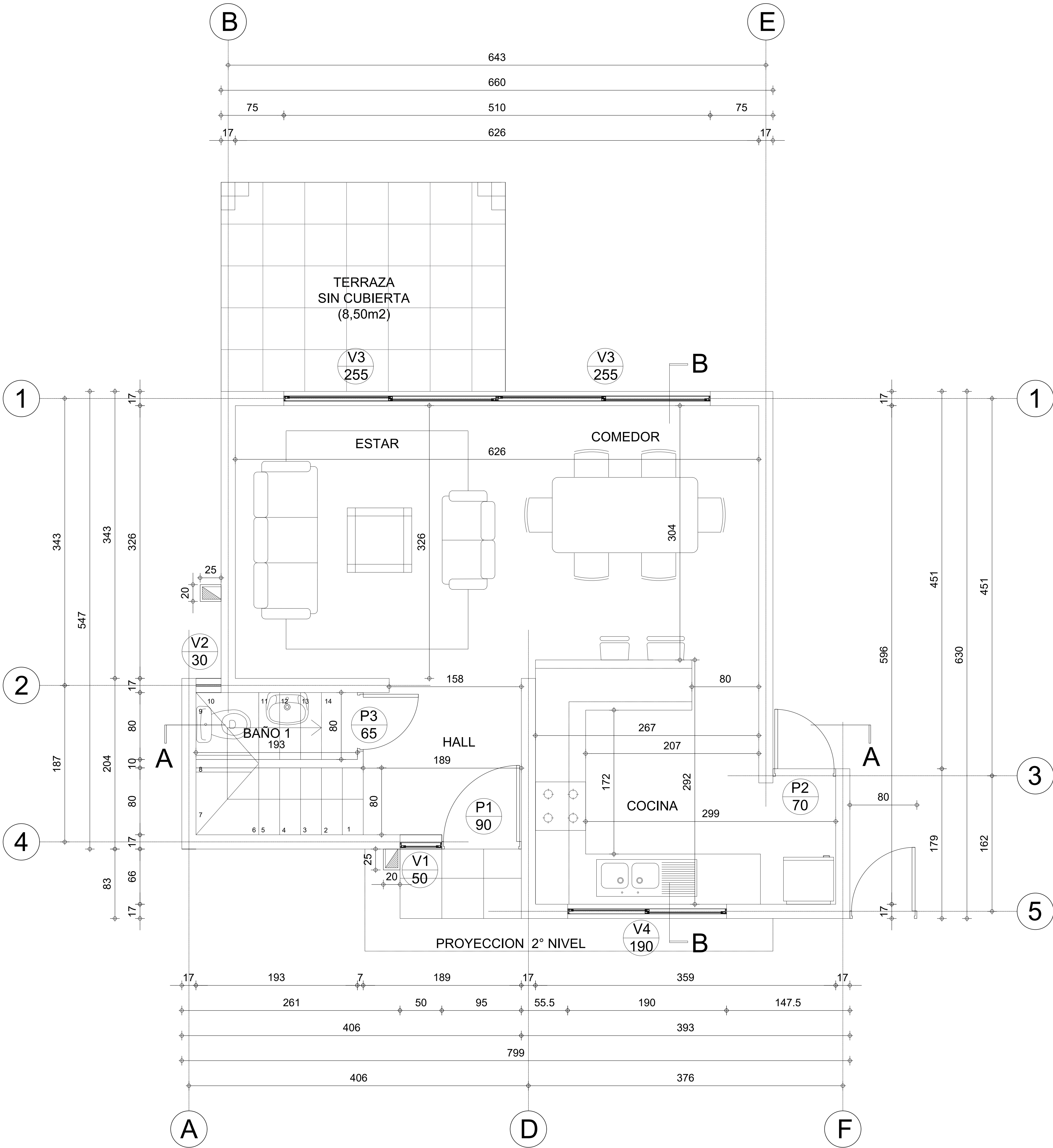
PLANTA PRIMER PISO ESCALA 1:50
